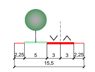
POPREČNI PRESJEK B - B
