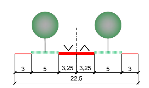
POPREČNI PRESJEK A - A
