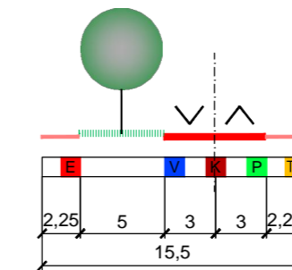
POPREČNI PRESJEK B - B
