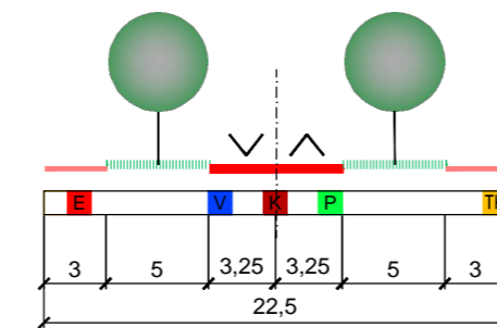
POPREČNI PRESJEK A - A
